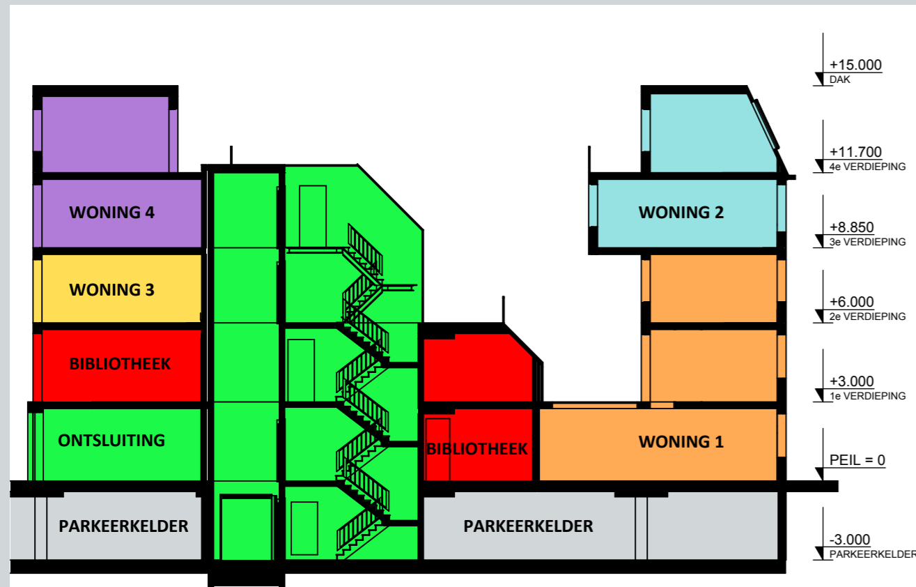
DOORSNEDEN AA
